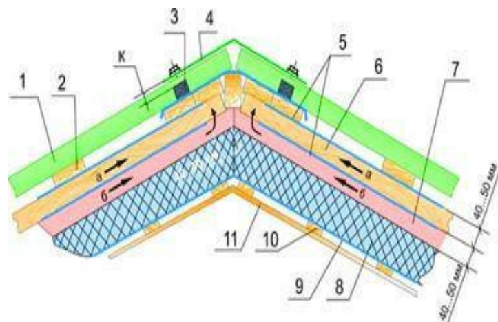
Рис.5 Утепление кровли
